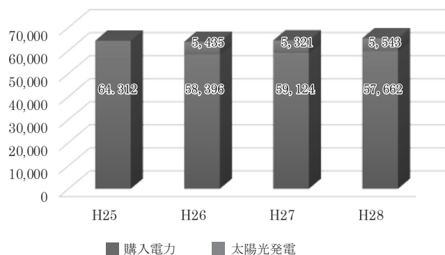
藤里中学校電気使用状況
